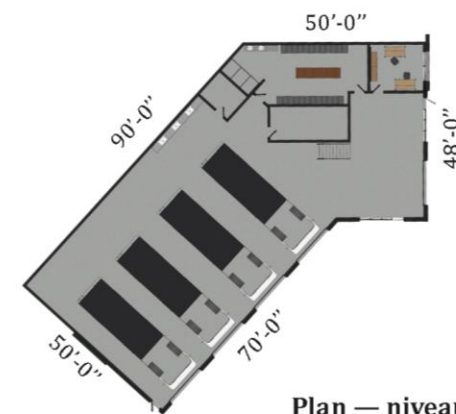
Plan — niveau 0
